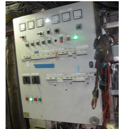
© / Fondation Tara Océan Tableau de distribution 230V alternatif.
