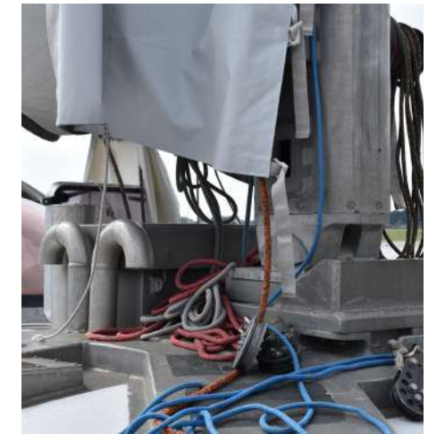
© Caroline Ovia / Fondation Tara Océan Tuyaux de sortie de l'air de la salle des machines sur le pont au niveau du pied de mât de misaine.
